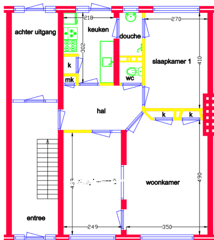
beganegrond
