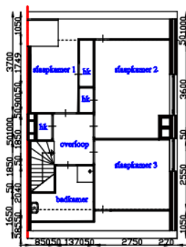
Verdieping
