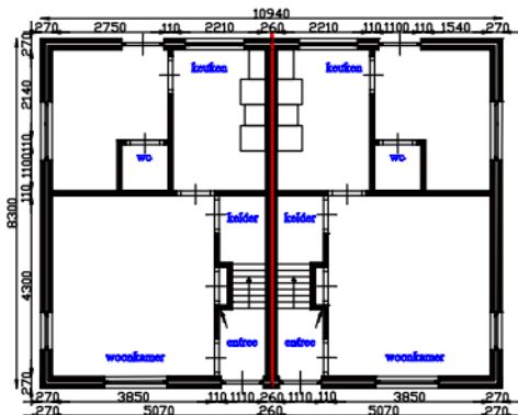
Begane grond
