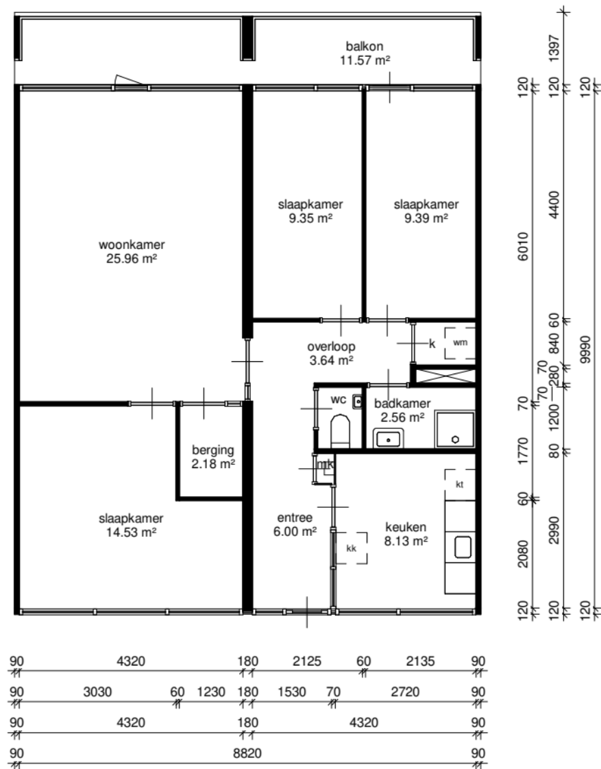
eerste verdieping
