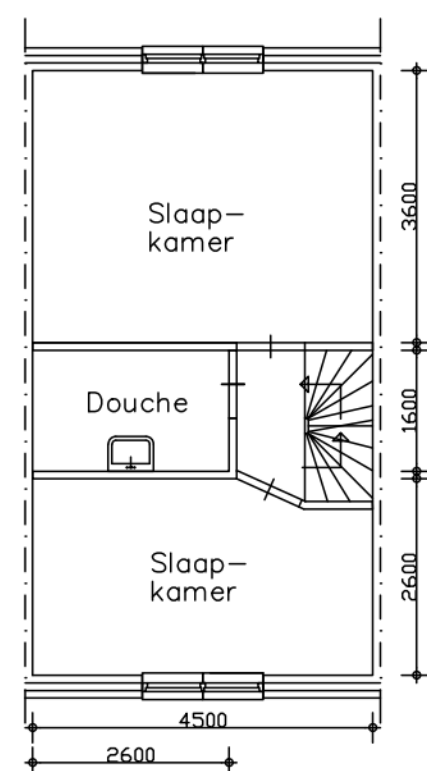
Verdieping
