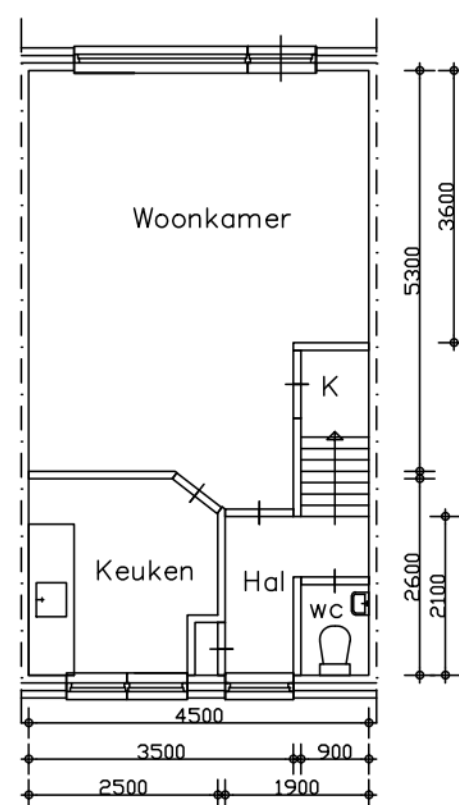
Beganegrond
