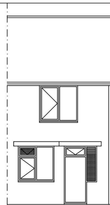
Voorgevel
