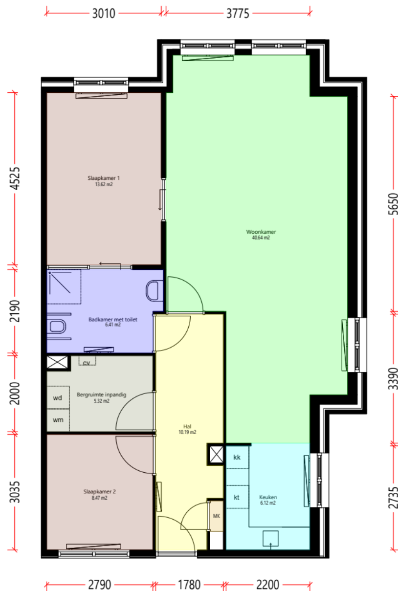
Verdieping_2e
