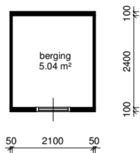
begane grond
