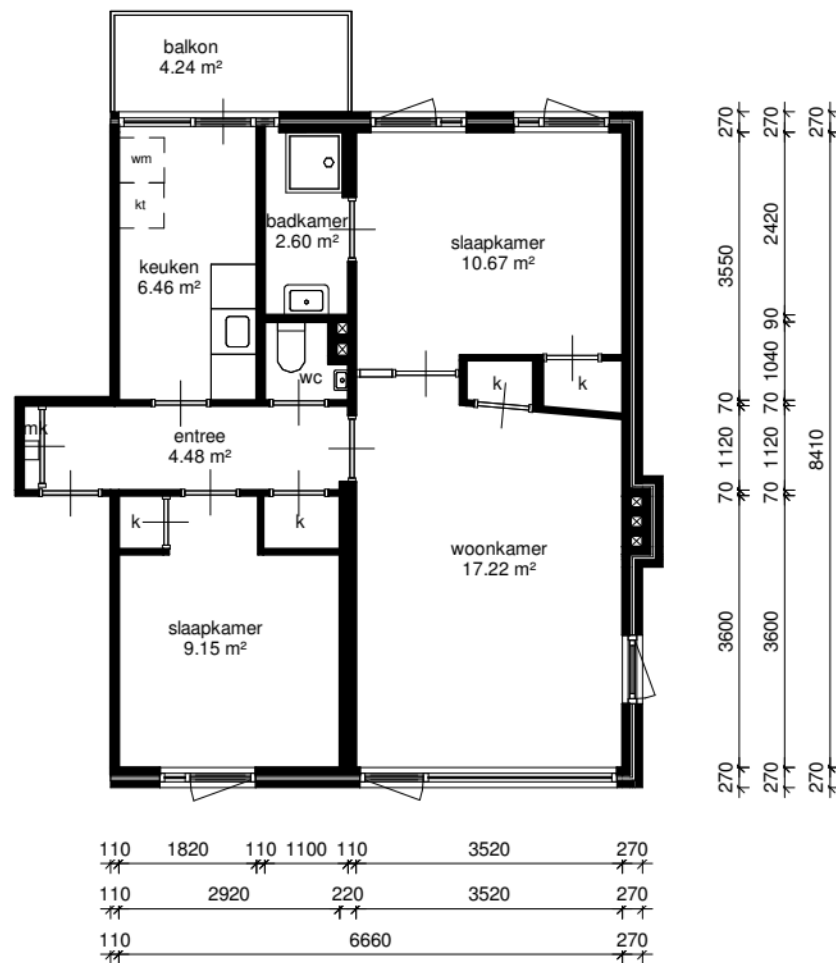
eerste verdieping
