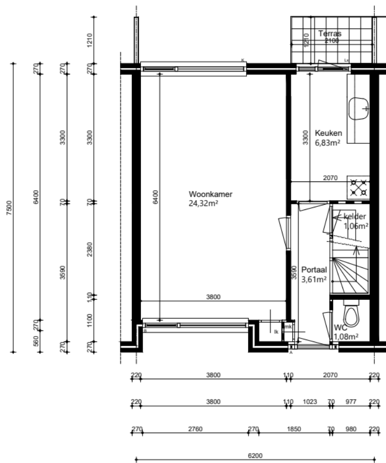
Begane grond
