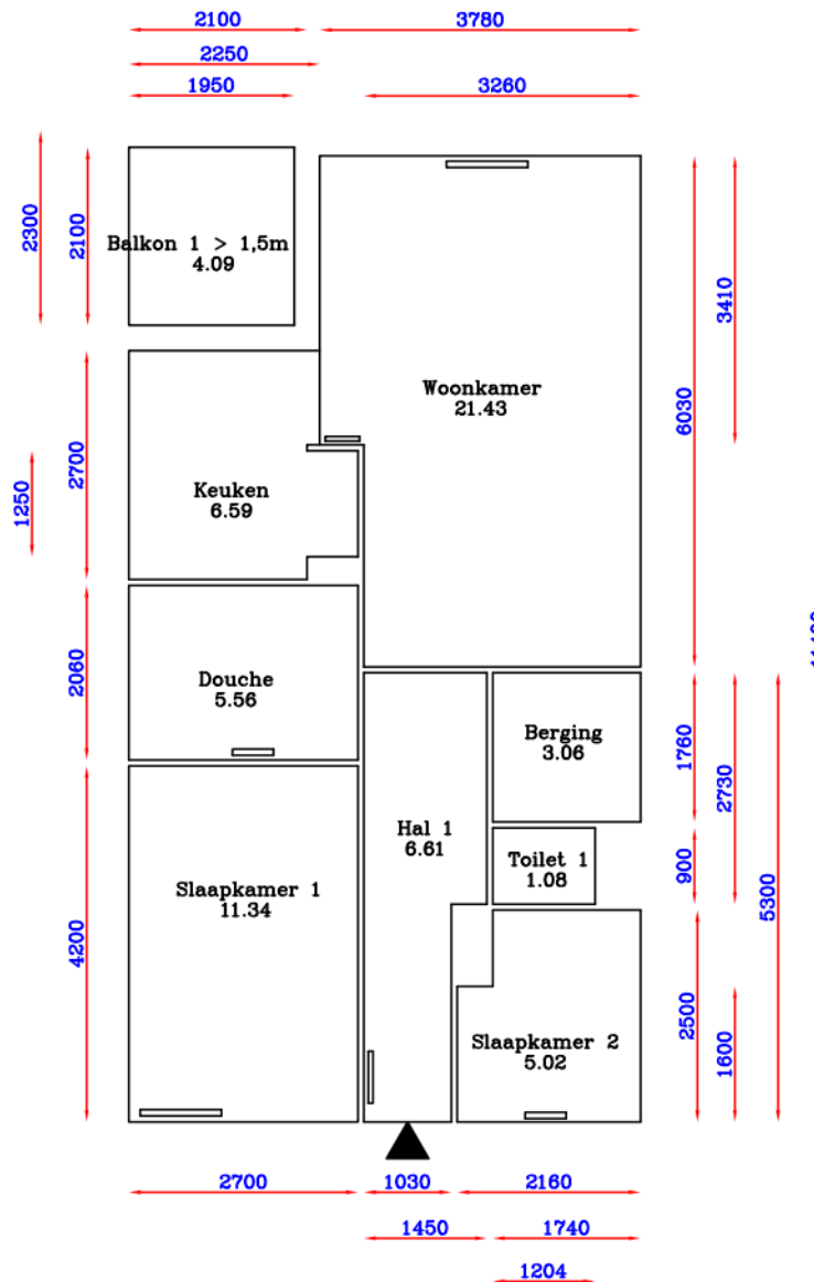
2e Verdieping
