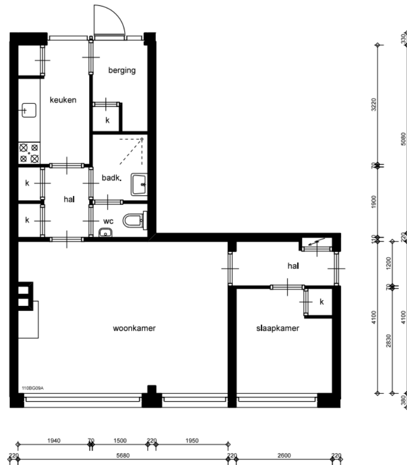
BEGANE GROND
