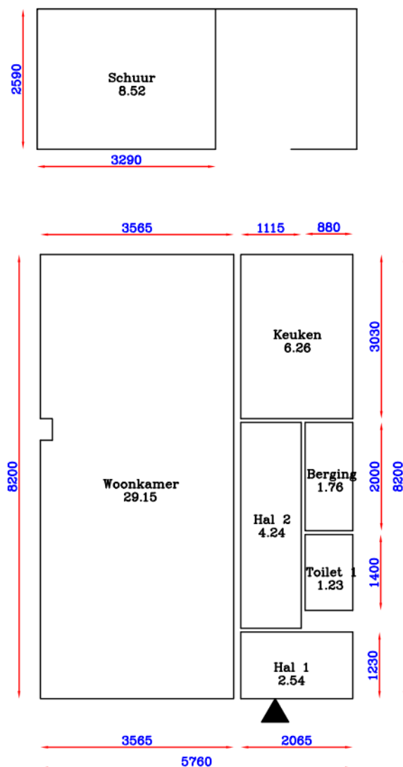
Begane grond
