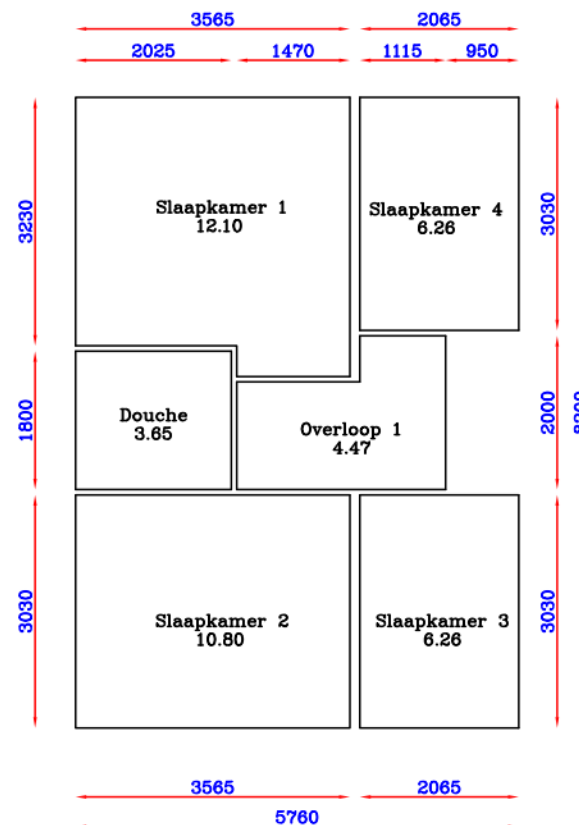
1e Verdieping
