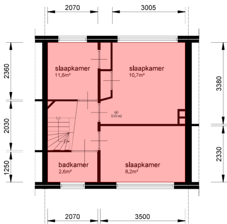
Verdieping_1e
