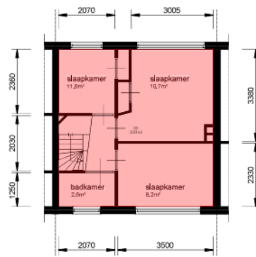
Verdieping_1e
