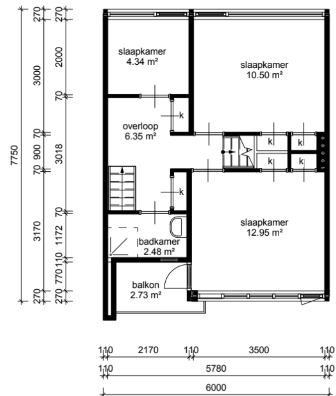
Eerste Verdieping GBO: 40.99m²
