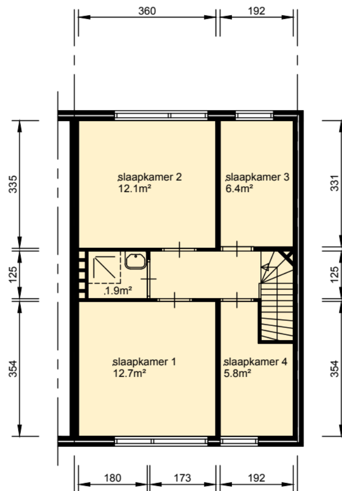
verdieping
