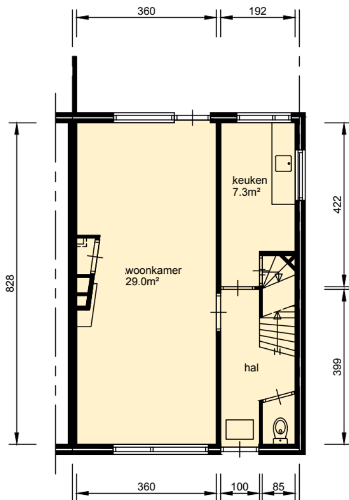
begane grond
