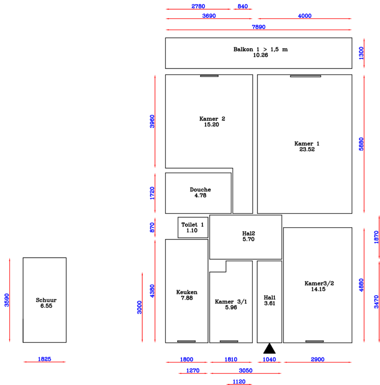
Begane grond
