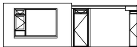
Achtergevel
