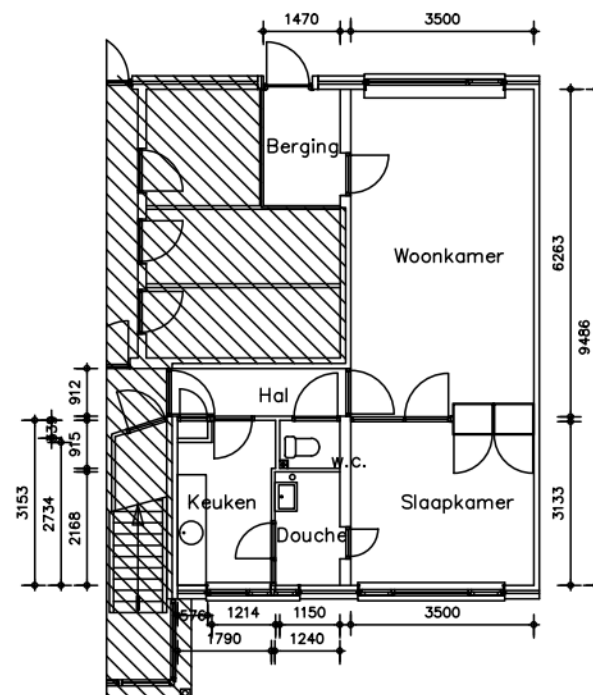
Begane grond
