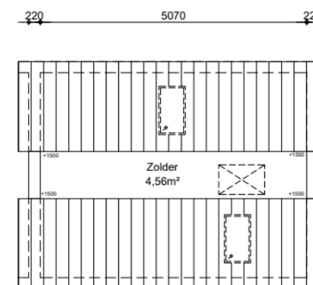
2e verdieping GO wonen 4,56m²
