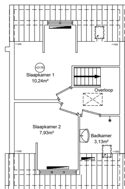
1e verdieping GO wonen 27,21m²
