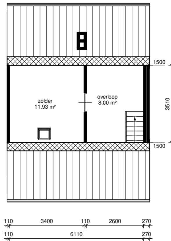
eerste verdieping
