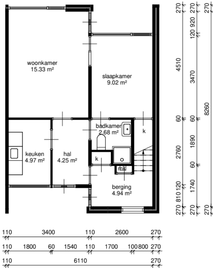
begane grond
