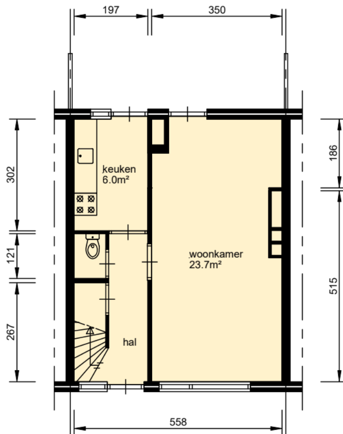
begane grond
