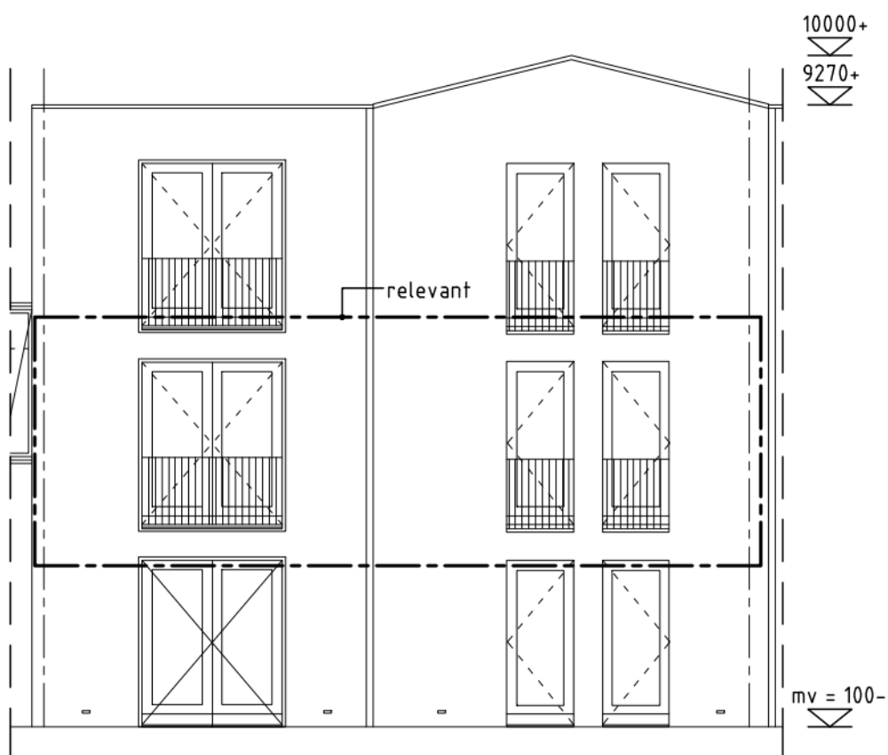
Achtergevel
