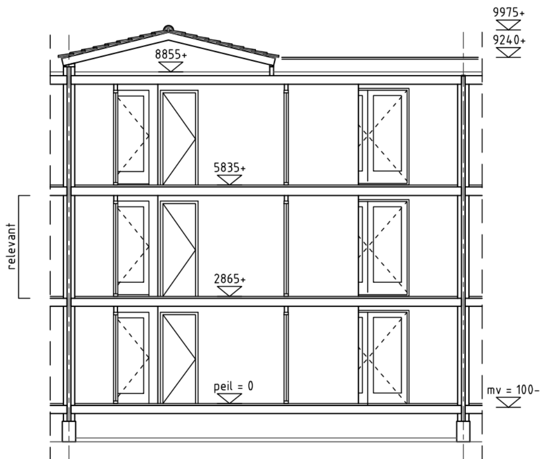
Doorsnede
