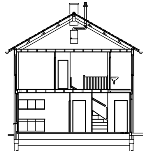
Doorsnede
