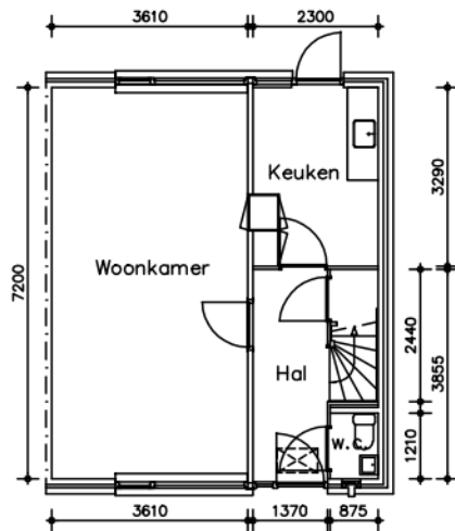
Begane grond
