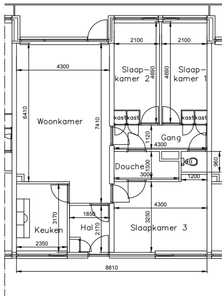
Plattegrond
