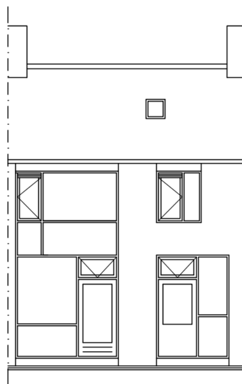
Achtergevel
