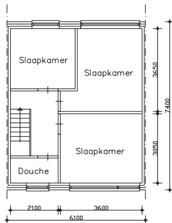
Verdieping
