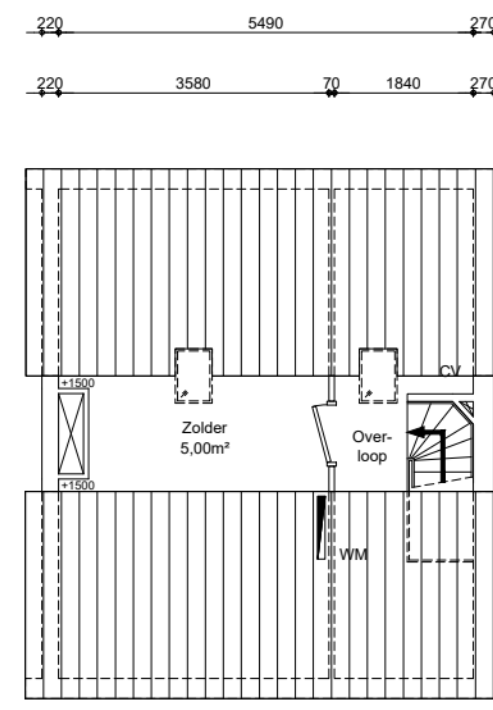
2e verdieping GO wonen 8,40m²
