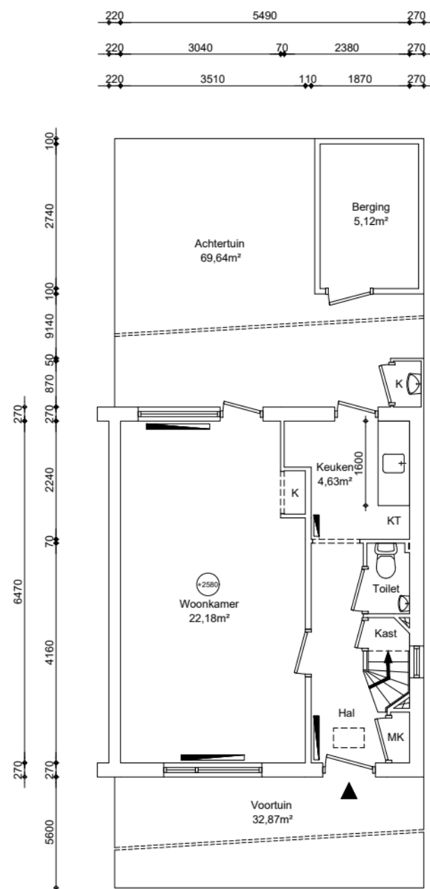
Begane grond GO wonen 35,52m²
