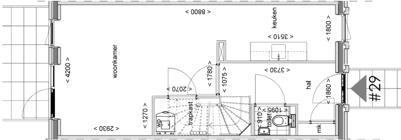
Begane grond
