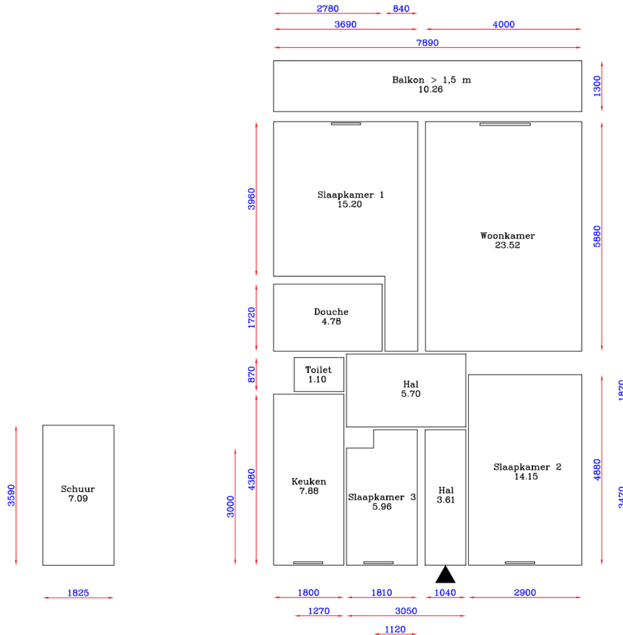
Begane grond
