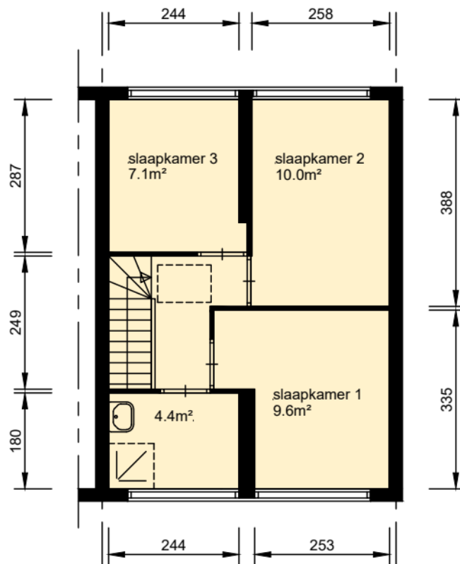
verdieping
