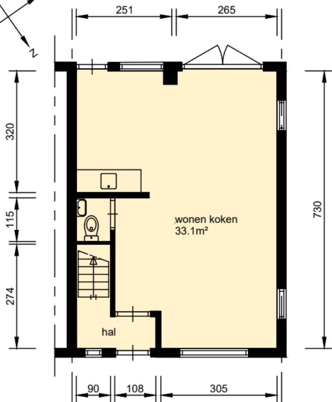
begane grond
