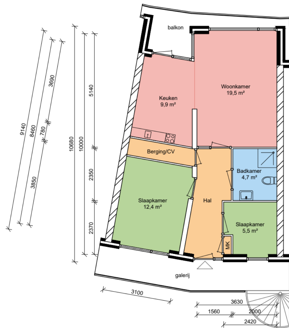
2e Verdieping
