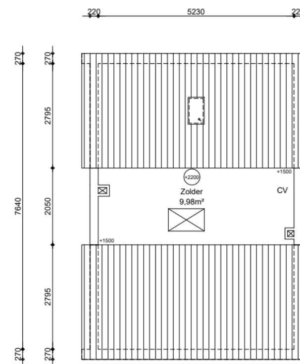
2e verdieping GO wonen 0,00m²
