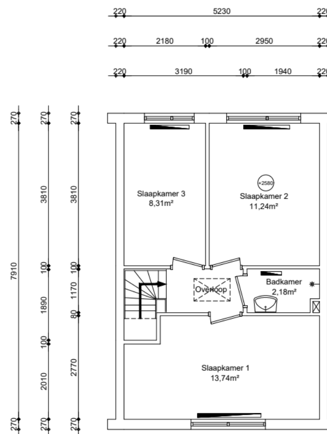
1e verdieping GO wonen 41,37m²
