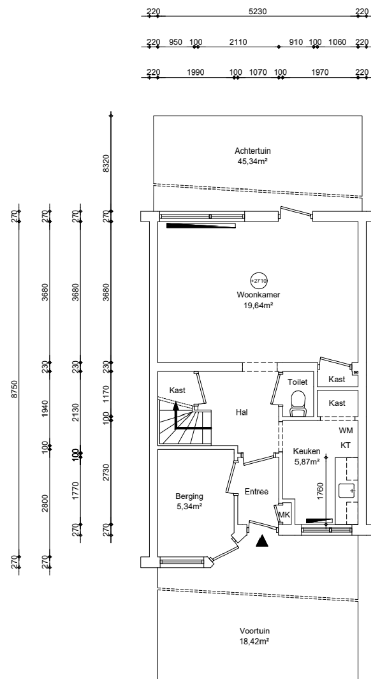
Begane grond GO wonen 41,61m²
