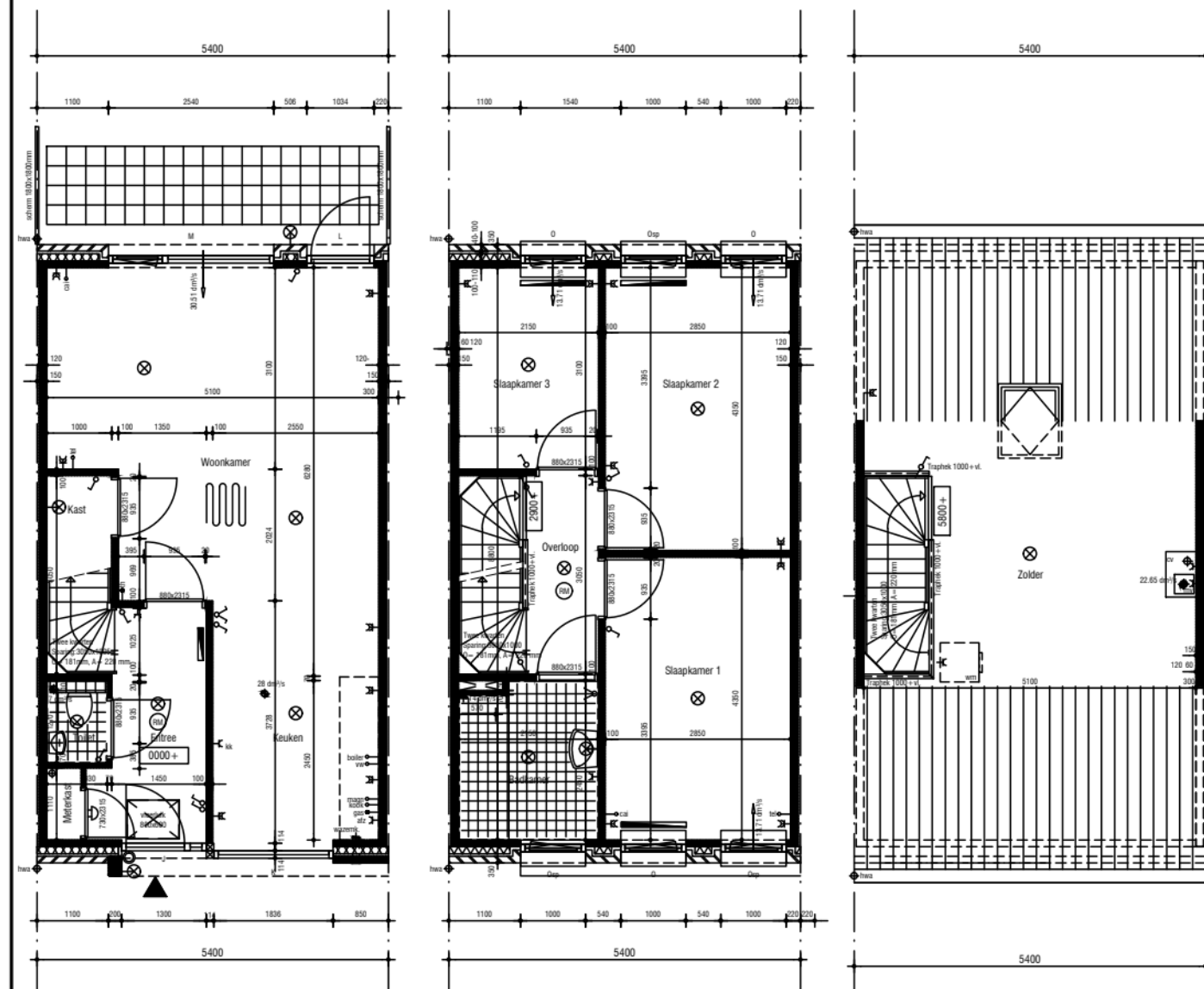
BEGANE GROND
