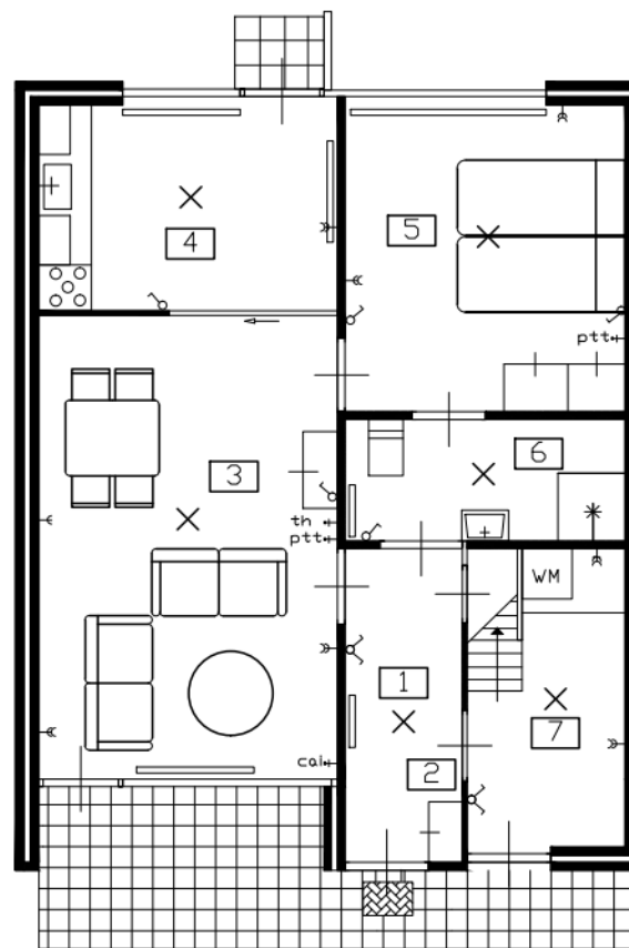
BEGANE GROND
