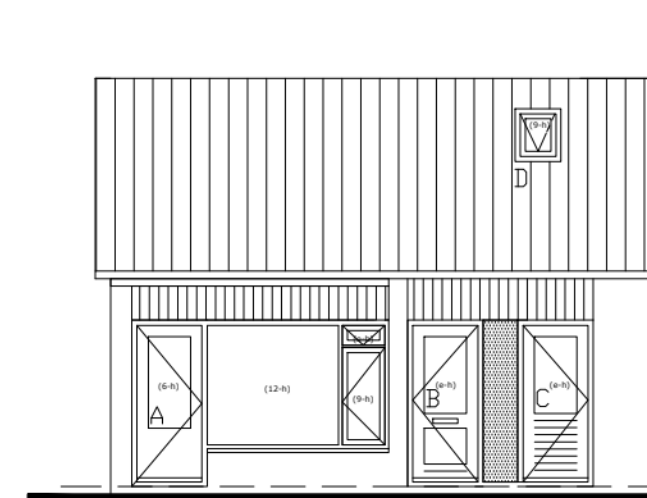
VOORGEVEL
