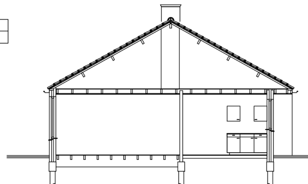
Doorsnede
