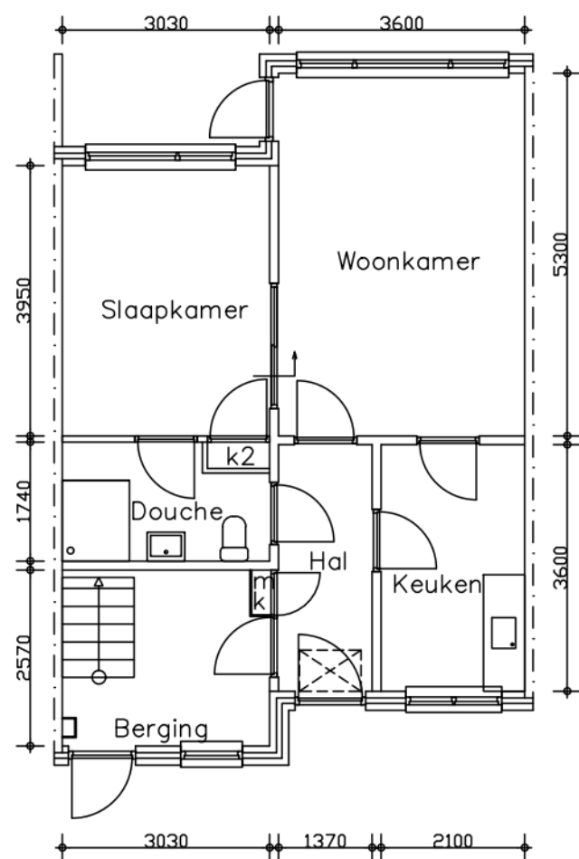
Begane grond
