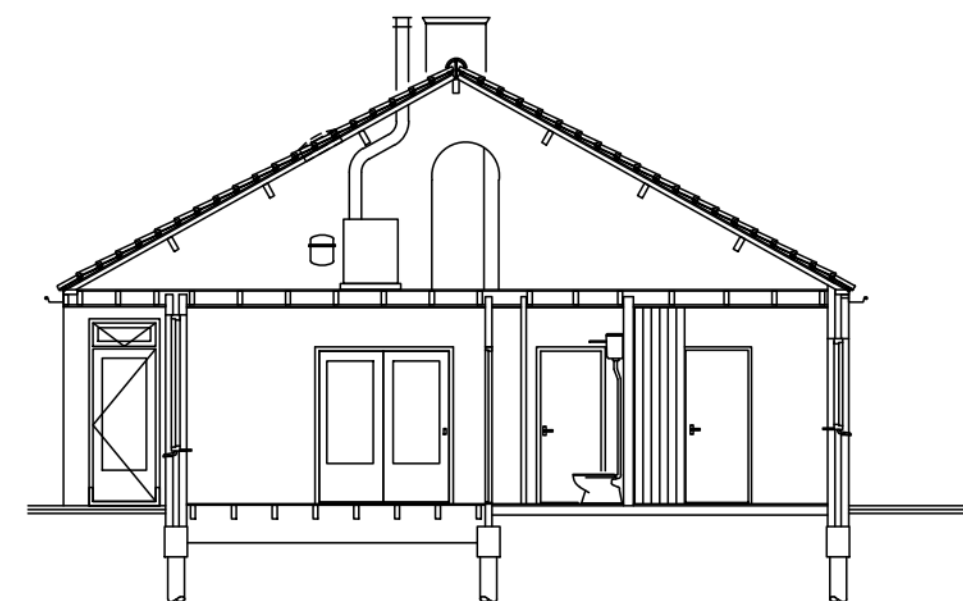
Doorsnede
