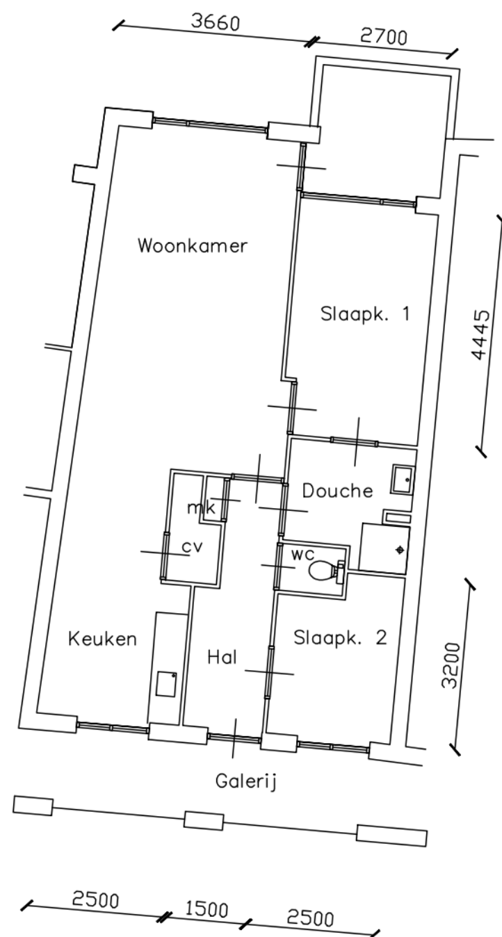
1e Verdieping
