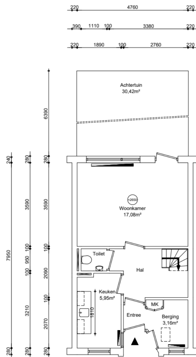
Begane grond GO wonen 36,73m²
