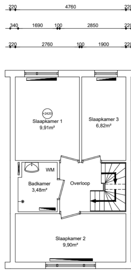
1e verdieping GO wonen 37,57m²
