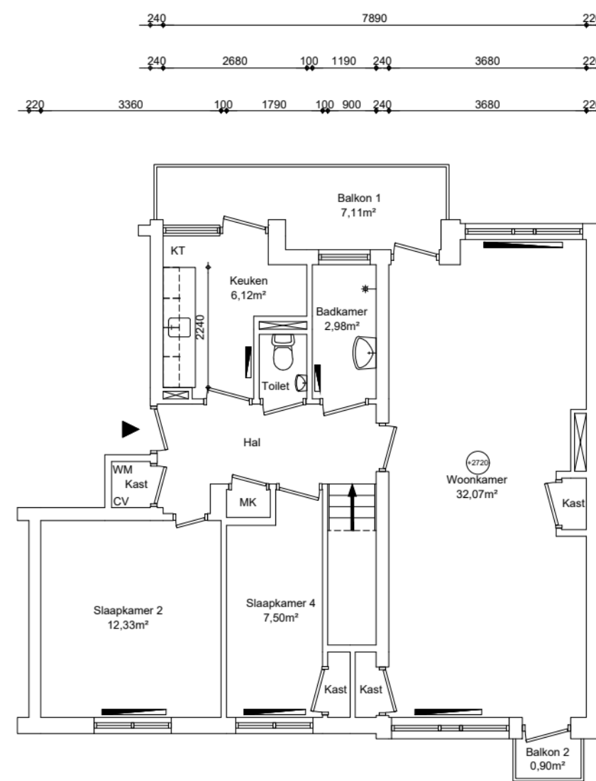
1e verdieping GO wonen 76,04m²
