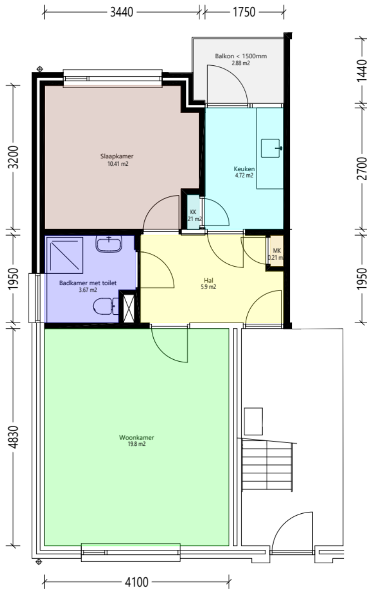
Verdieping_1e
