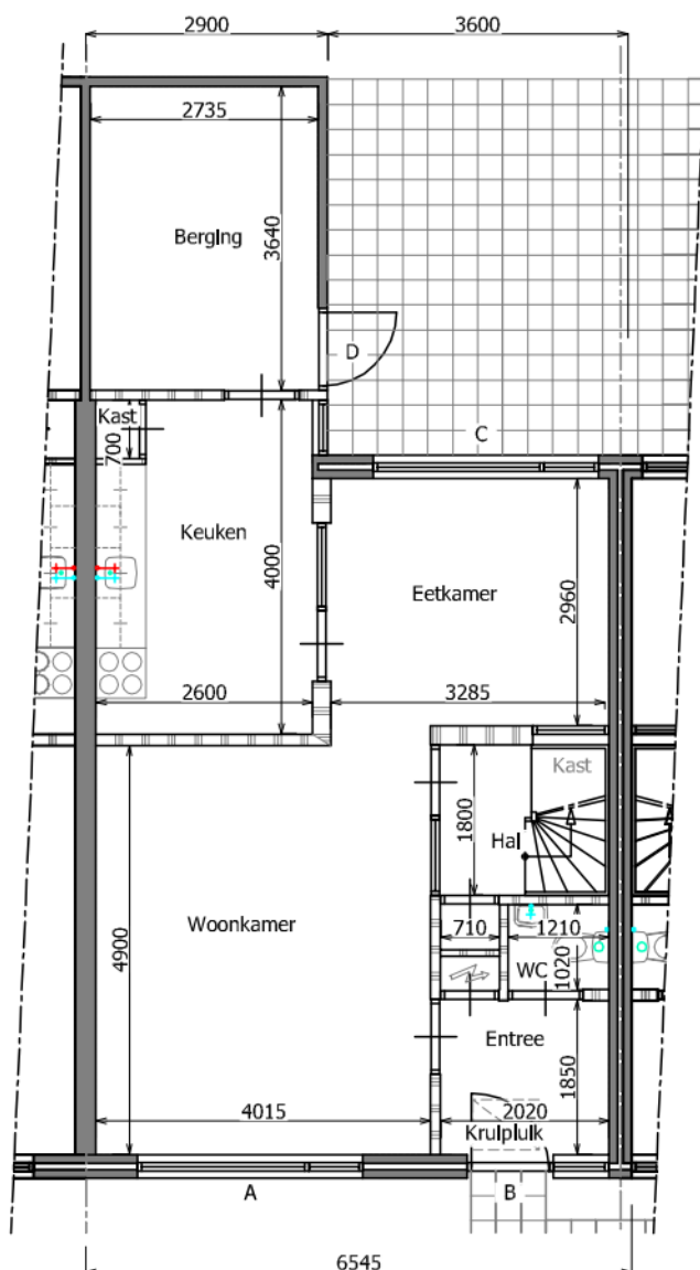
Begane grond
