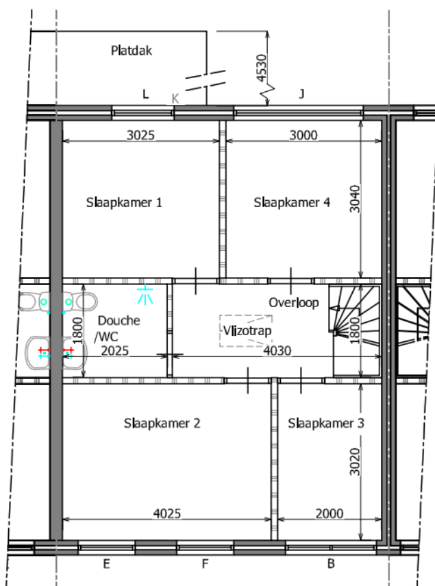
1e verdieping
