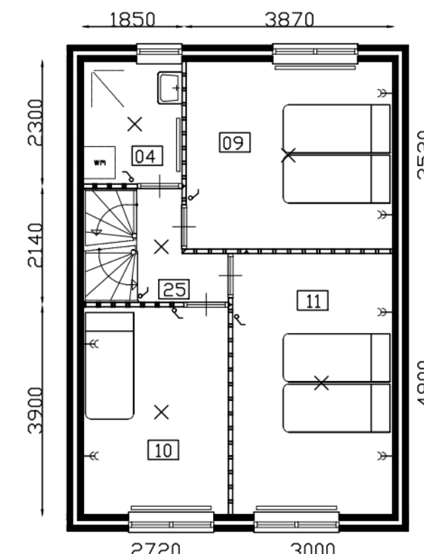
EERSTE VERDIEPING
