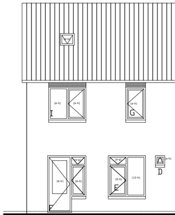
ACHTERGEVEL
