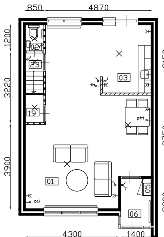
BEGANE GROND
