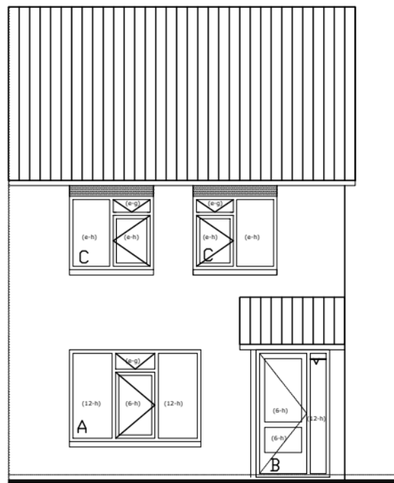
VOORGEVEL
