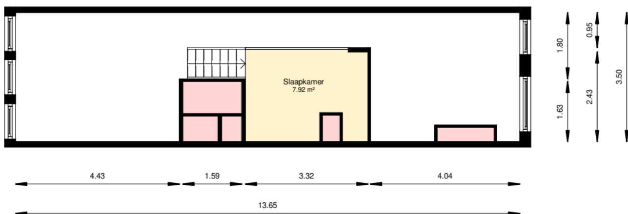
01 Eerste verdieping
