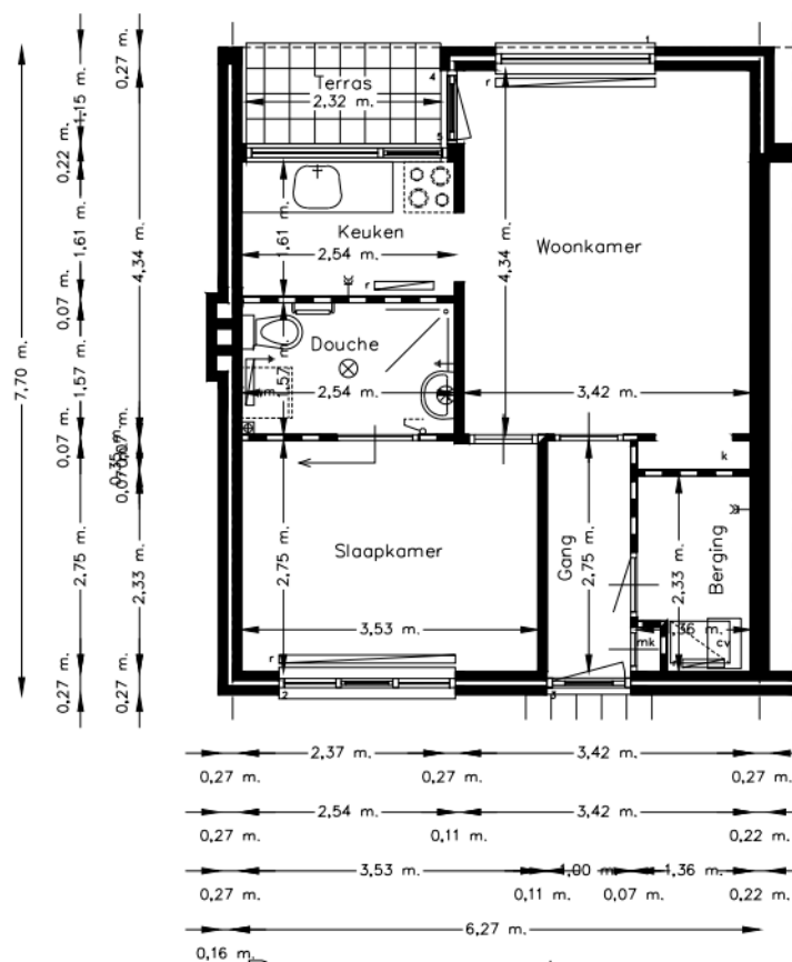
Begane grond
