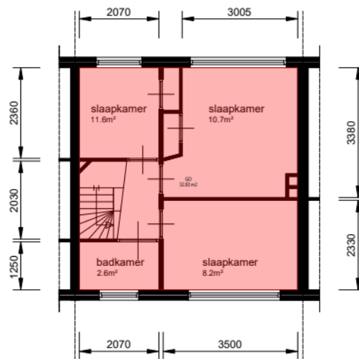
Verdieping_1e
