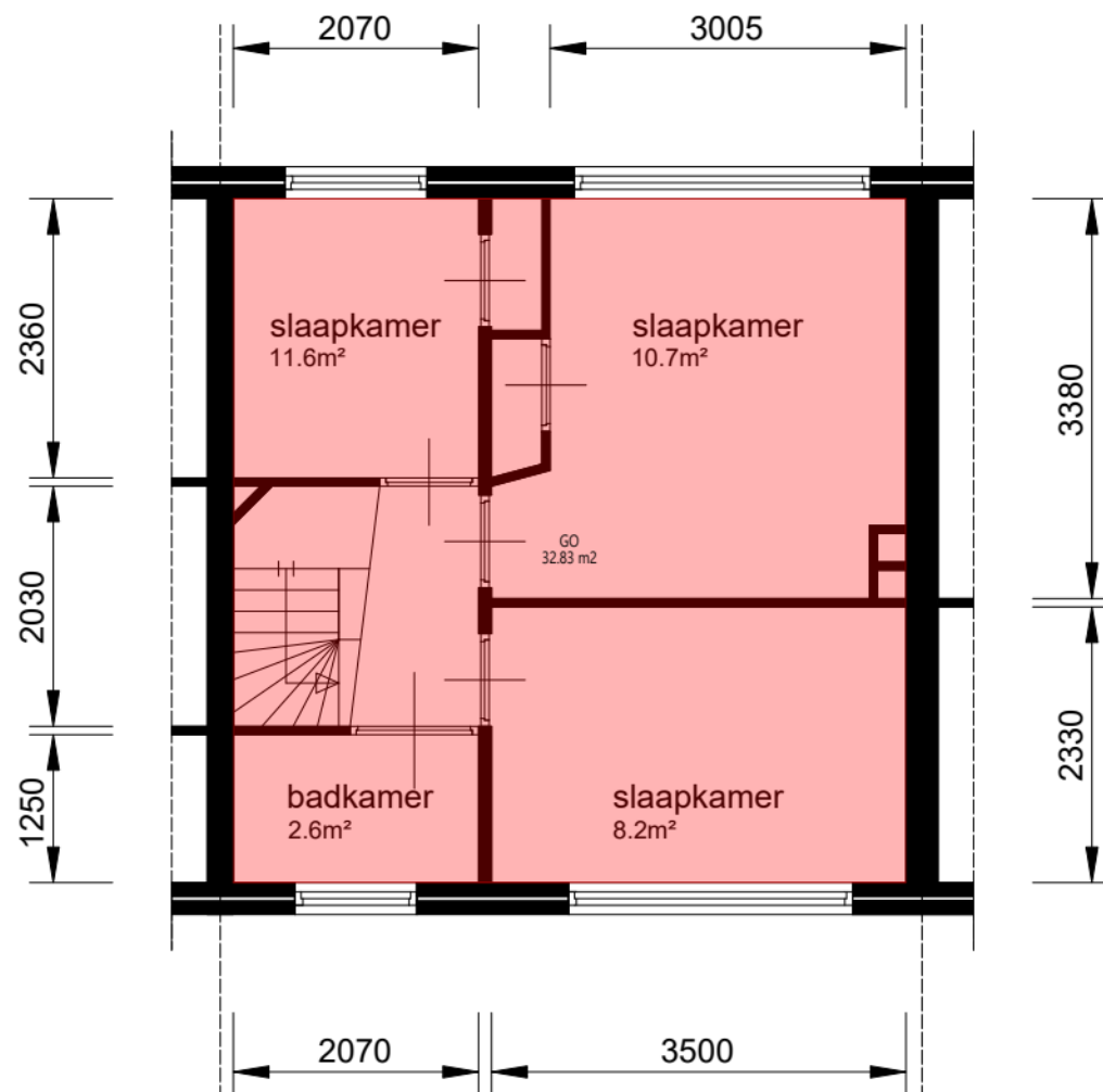
Verdieping_1e
