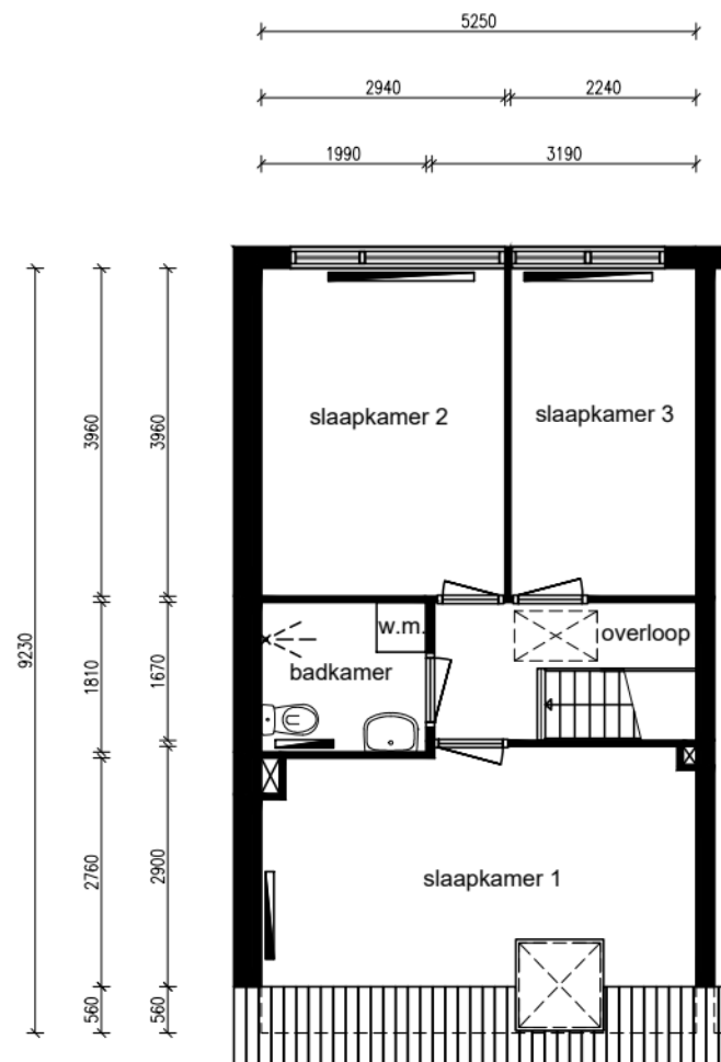
1e verdieping
