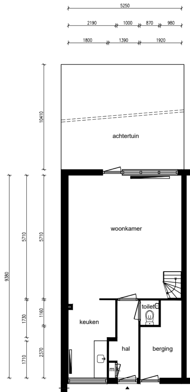
Begane grond
