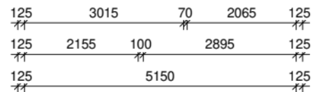
eerste verdieping
