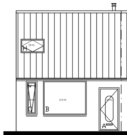
VOORGEVEL
