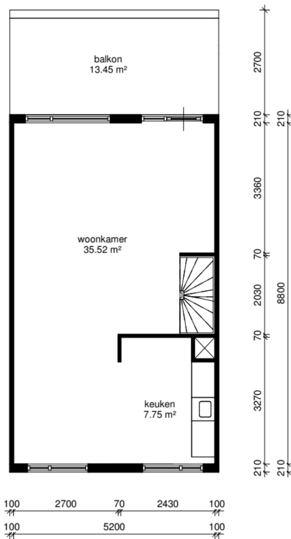
tweede verdieping
