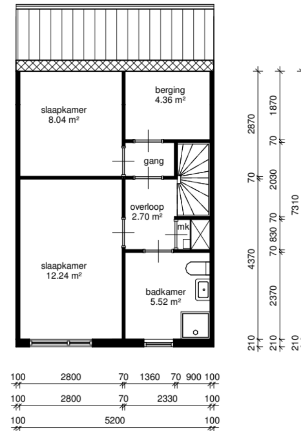
derde verdieping
