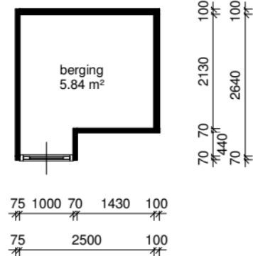
begane grond
