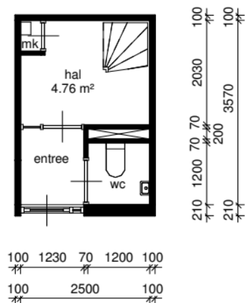
eerste verdieping
