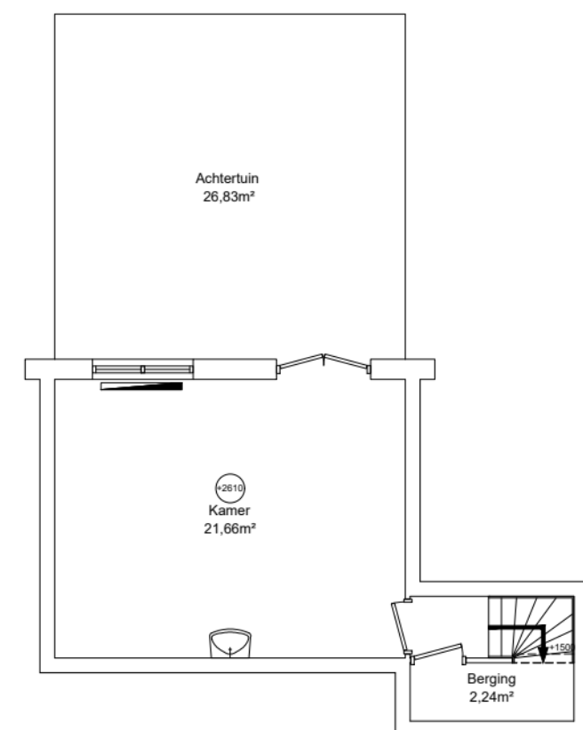
Begane grond GO wonen 26,26m²
