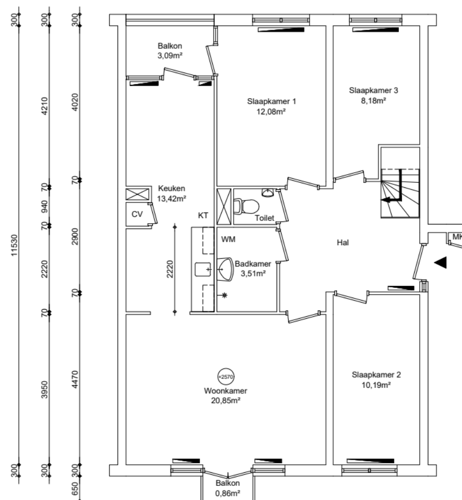
1e verdieping GO wonen 83,55m²
