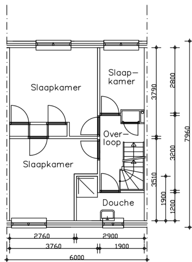
1e Verdieping
