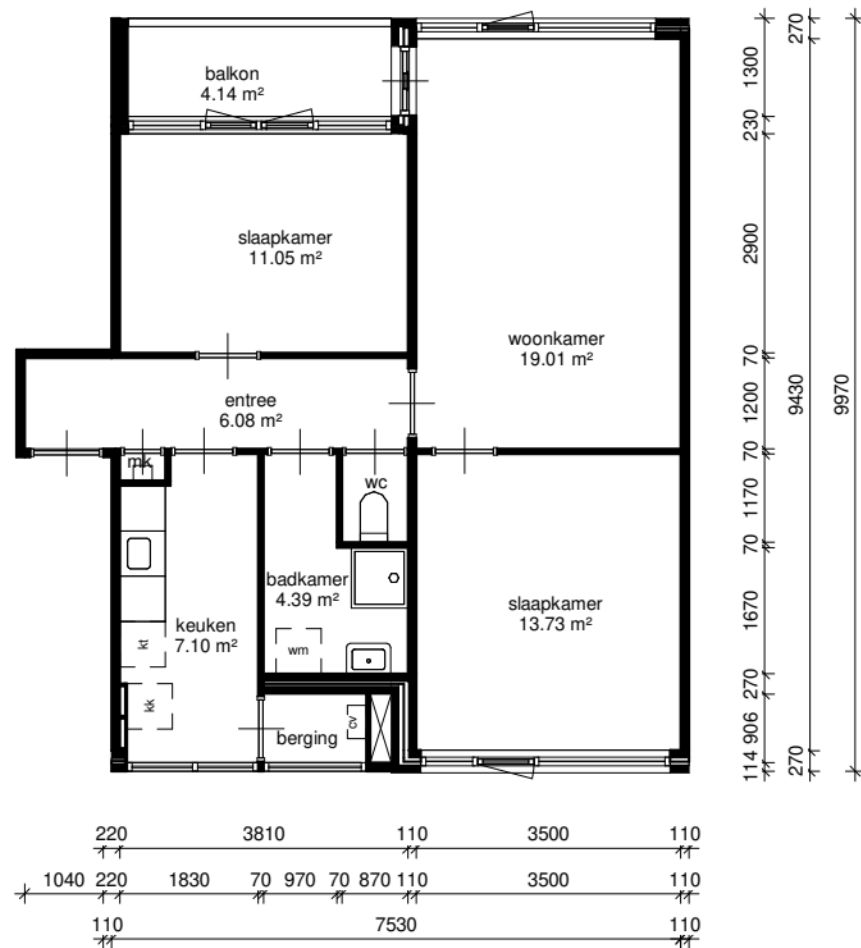
eerste verdieping
