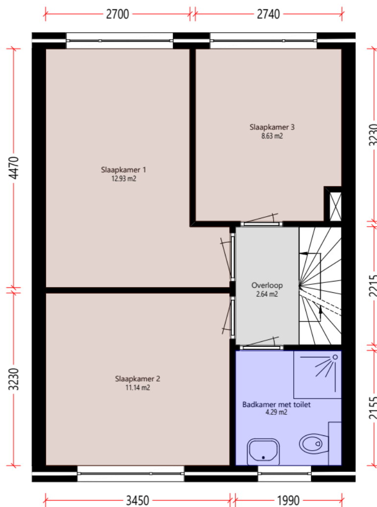
Verdieping_1e
