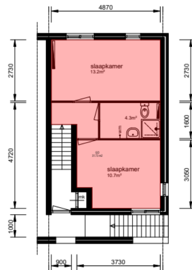
Verdieping_1e
