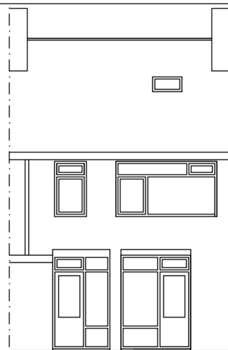
Achtergevel
