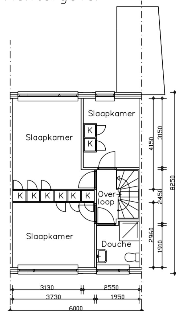
Verdieping
